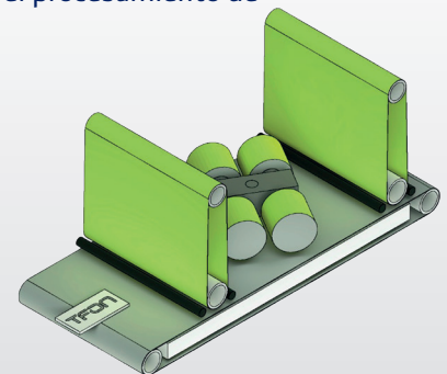
Ejemplo de estructura modular con 3 módulos: 2 desbarbado, 4 Redondeado de cantos y 5 satinado
