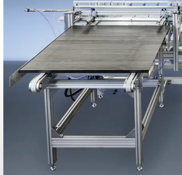
WKF 170 como instalación de biselado automática con módulo de avance y mesa de rodillos
