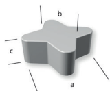
Star (STE)
